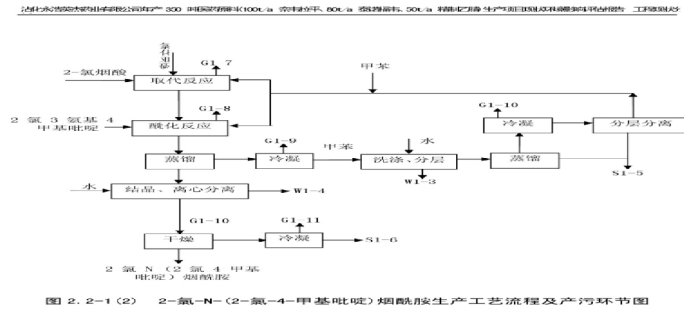
图 2.2-1 (2) 2-氯-N-(2-氯-4-甲基吡啶)烟酰胺生产工艺流程及产污环节图
