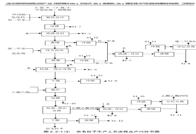
图 2.2-1 (3) 奈韦拉平生产工艺流程及产污环节图
